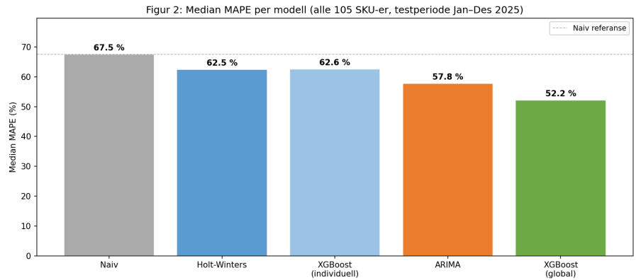
Figur 2: Median MAPE per modell — sammenligning av prognosemodeller i testperioden
